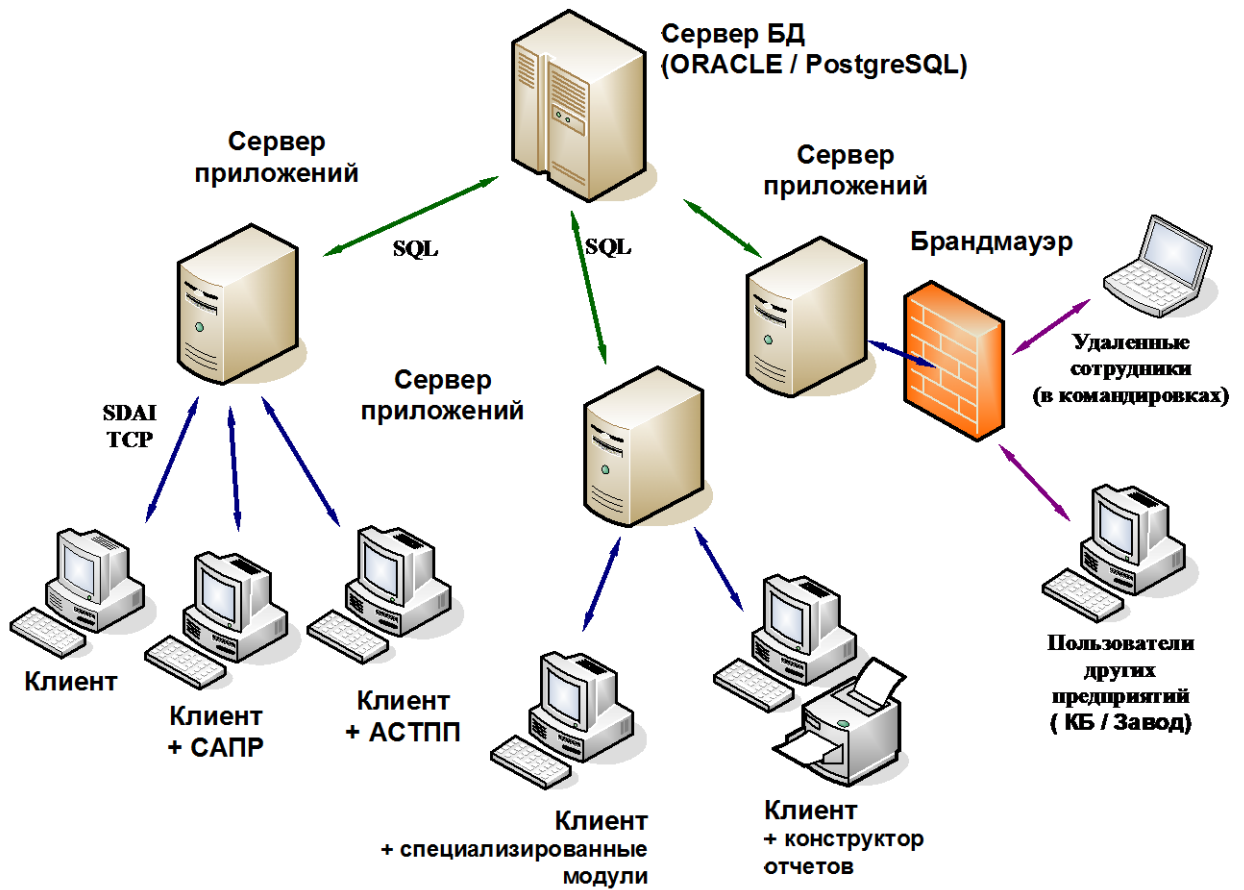
Рис. 1. Трехуровневая архитектура "Клиент-Сервер"
