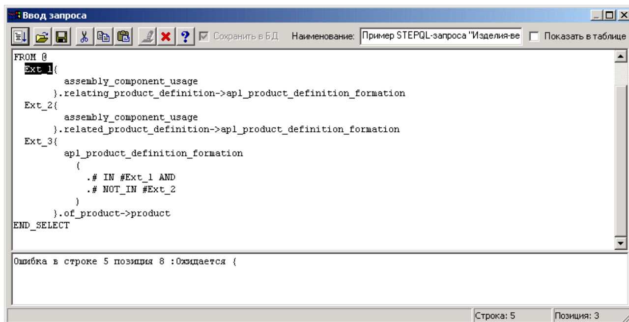
Рис. 22. Окно редактора запросов на языке STEPQL
