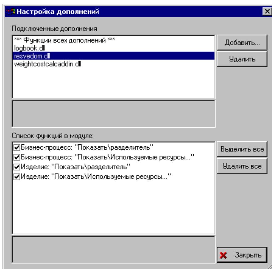
Рис. 27. Окно подключению модулей дополнения
