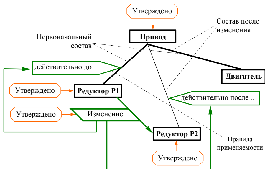
Рис. 12. Описание изменения структуры изделия в PSS
