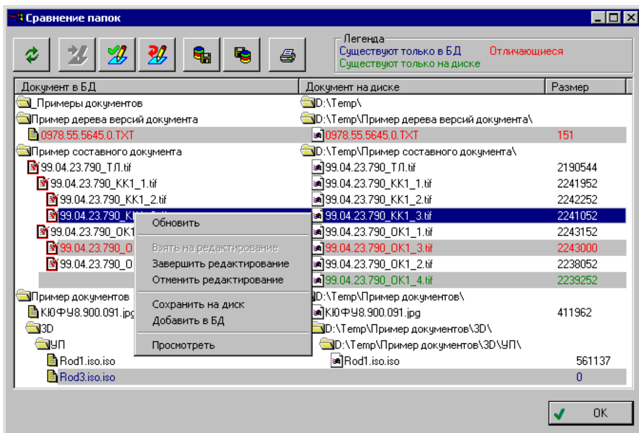
Рис. 6. Диалоговое окно сравнения документов в БД с файлами на диске
