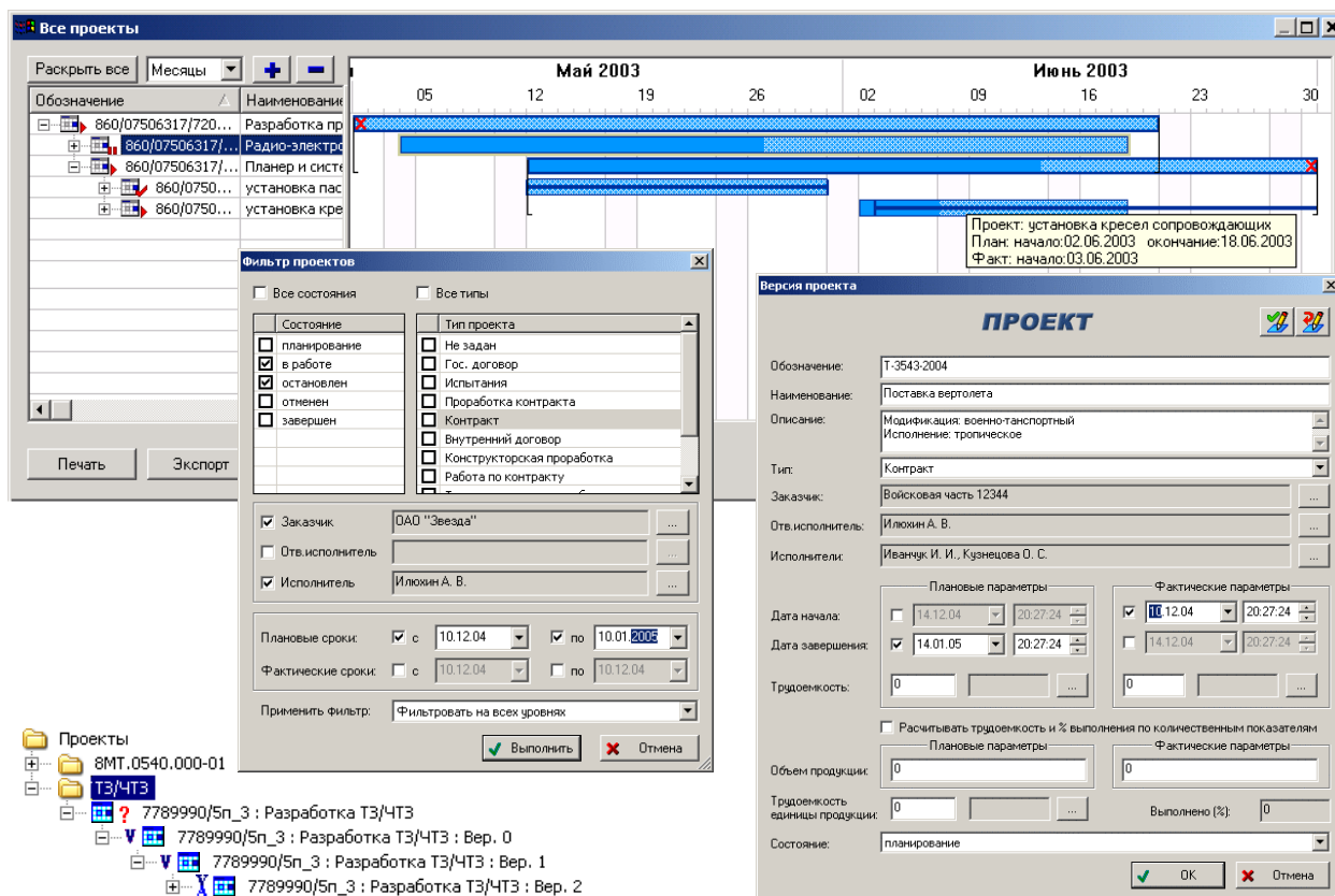
Рис. 25. Экранные формы управления проектами
