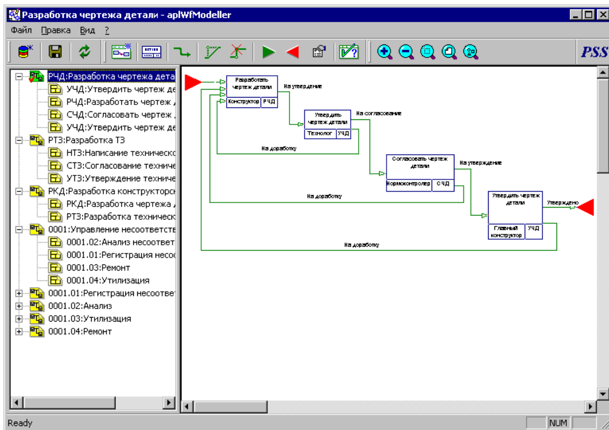
Рис. 24. Пример шаблона процесса
