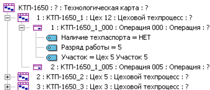
Рис. 10. Пример характеристик БП-операции
