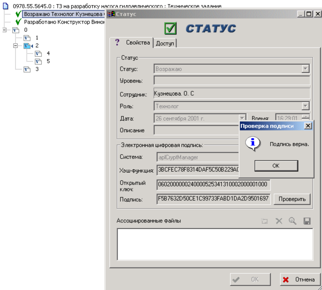
Рис. 4. Документ, его версии и статусы
