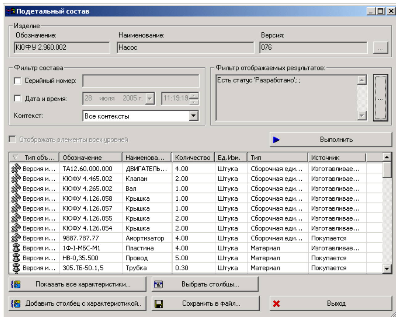
Рис. 2. Отчет - подетальный состав с фильтром
